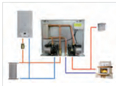
KIT Με ανοιχτό δοχείο διαστολής χωρίς ζεστό νερό χρήσης. KIT For open circuits without hot water supply.
