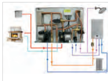
KIT Με ανοιχτό δοχείο διαστολής με ζεστό νερό χρήσης. KIT For open circuits with hot water supply.
